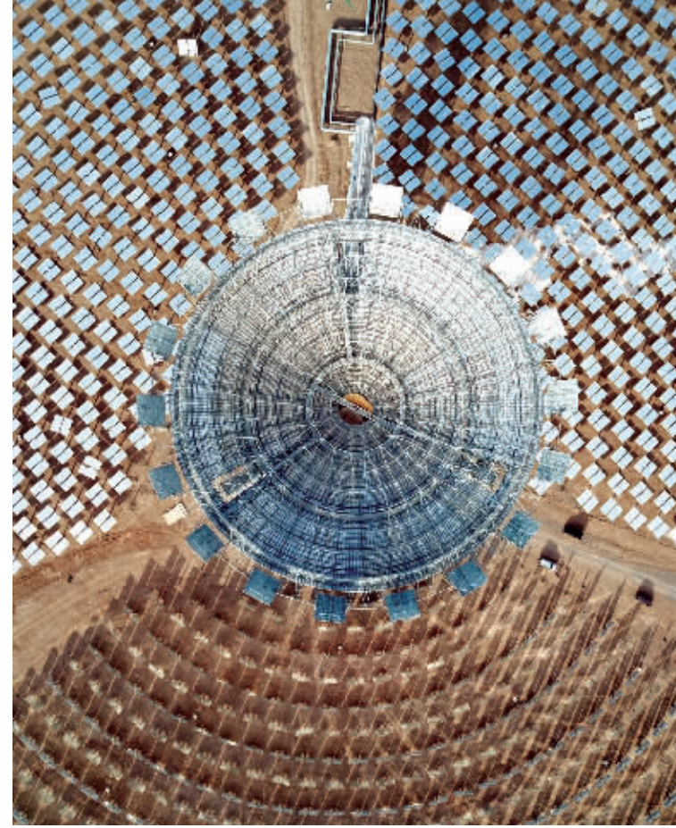
左图:甘肃玉门鑫能50兆瓦熔塔塔式光热电站 新华社图片 右图:隆基股份单晶电池生产工序 隆基股份供图 右图:川能动力盐边大面山风电项目 川能动力供图
