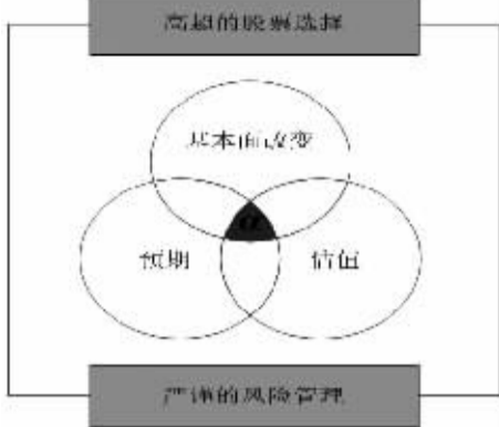
图2 选股模型
