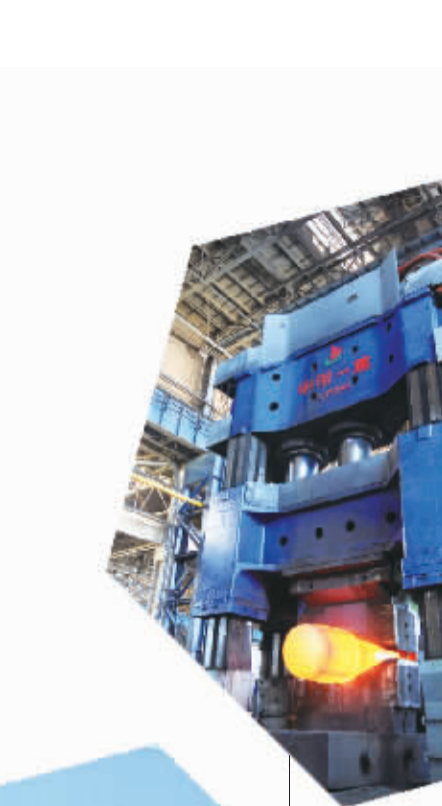
中国一重水压机锻造厂锻造活件现场
